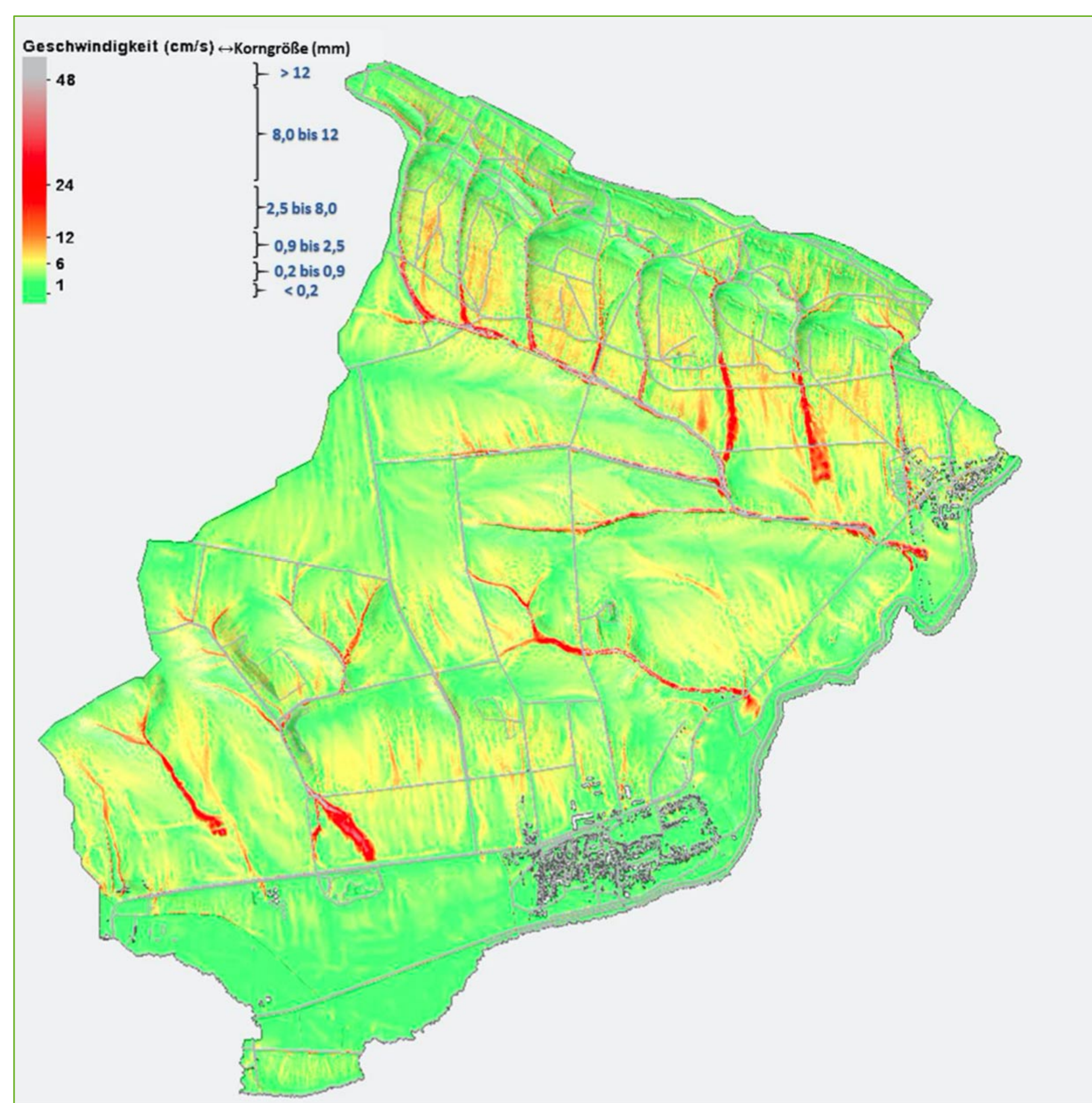
Hydrologische Untersuchungen von Keyline-Strukturen zeigen eine Reduzierung von 60 % der Bodenerosionen. Quelle: Tractebel Hydroprojekt GmbH
