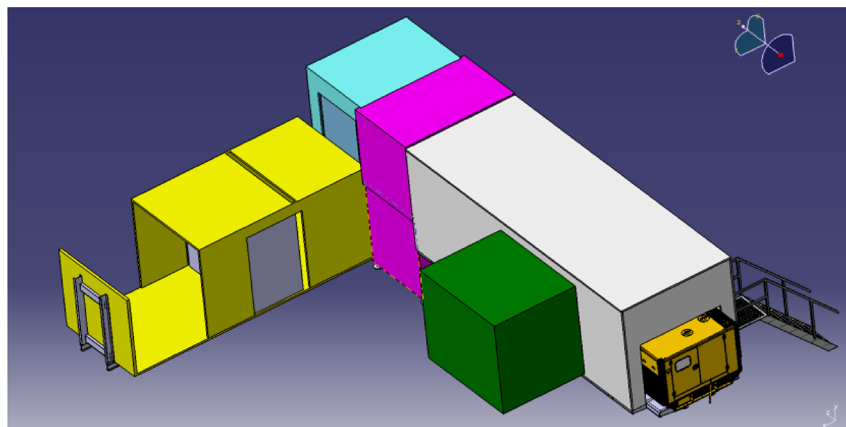
Abbildung (© Robby Tulke): Konstruktion mit Betäubungsbox (gelb) und Entblutebox (türkis) = Schwarzbereich Rind; Weißbereich Rind (pink), Weißbereich bzw. Verarbeitungsbereich (grau), wechselbare Kühlzellen (grün), Generator (gelb/schwarz)
