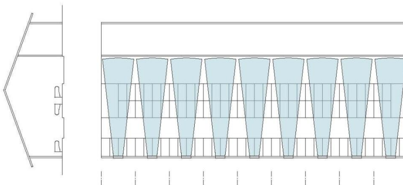
Abbildung 3: Anordnung von Ventilatoren in Querausrichtung
