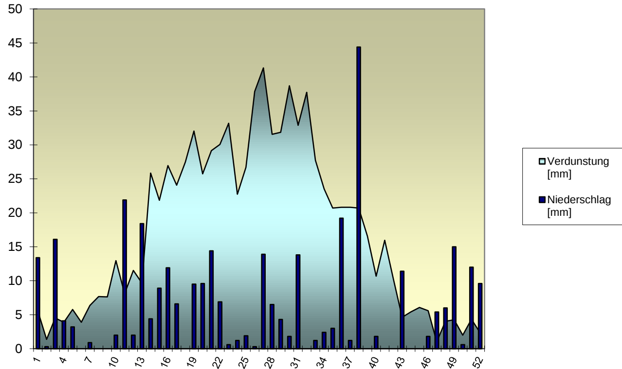
Niederschlag und Potentielle Verdunstung (nach Haude) 2018 893,94 mm pot. Verdunstung bei 335 mm Niederschlag
